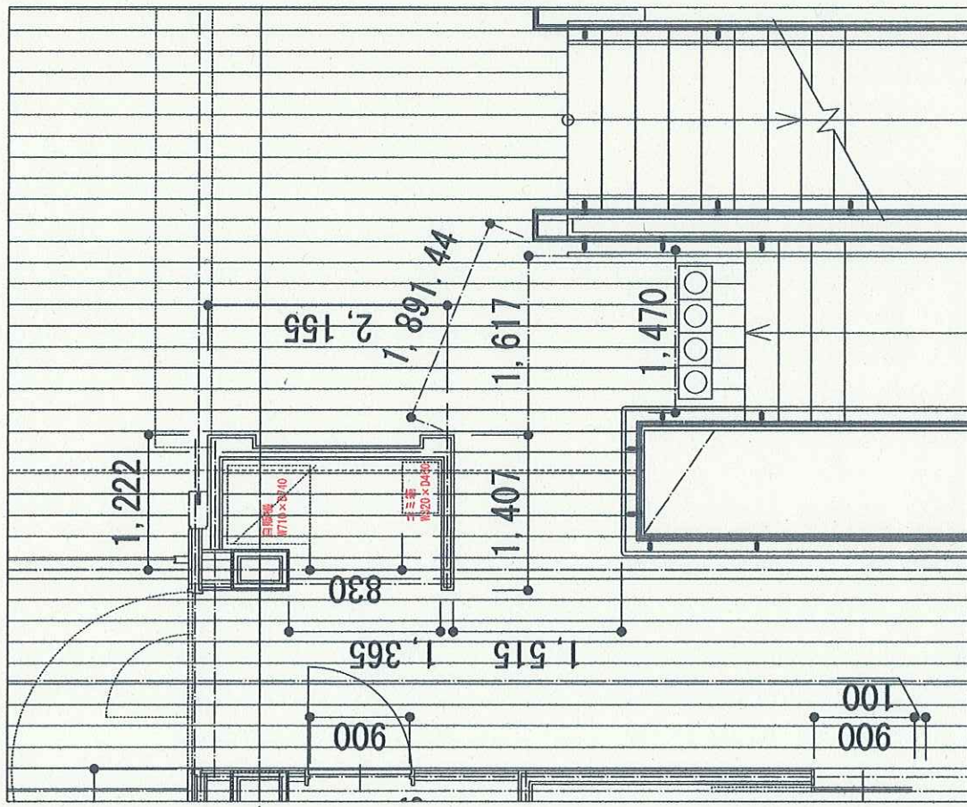
3階 ⑤18箱型タイプ
