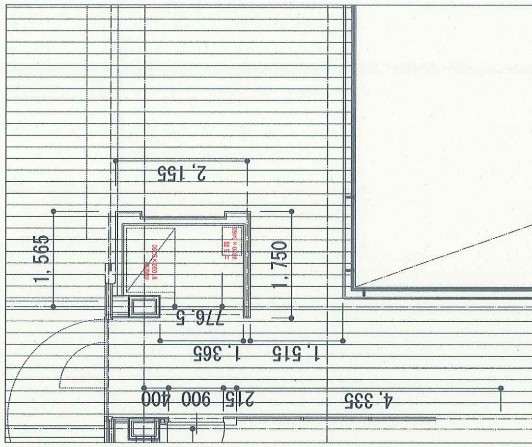
4階・5階 ⑩30箱型タイプ (平面は4階)
